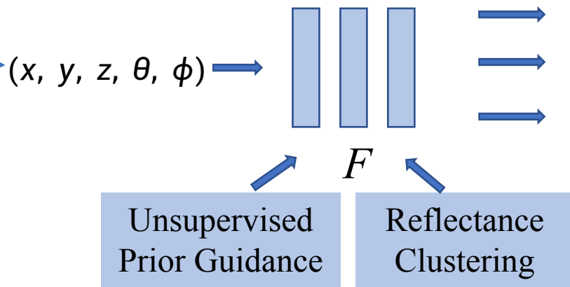
IntrinsicNeRF Framework
